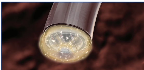
Tvorba plazmového pole
